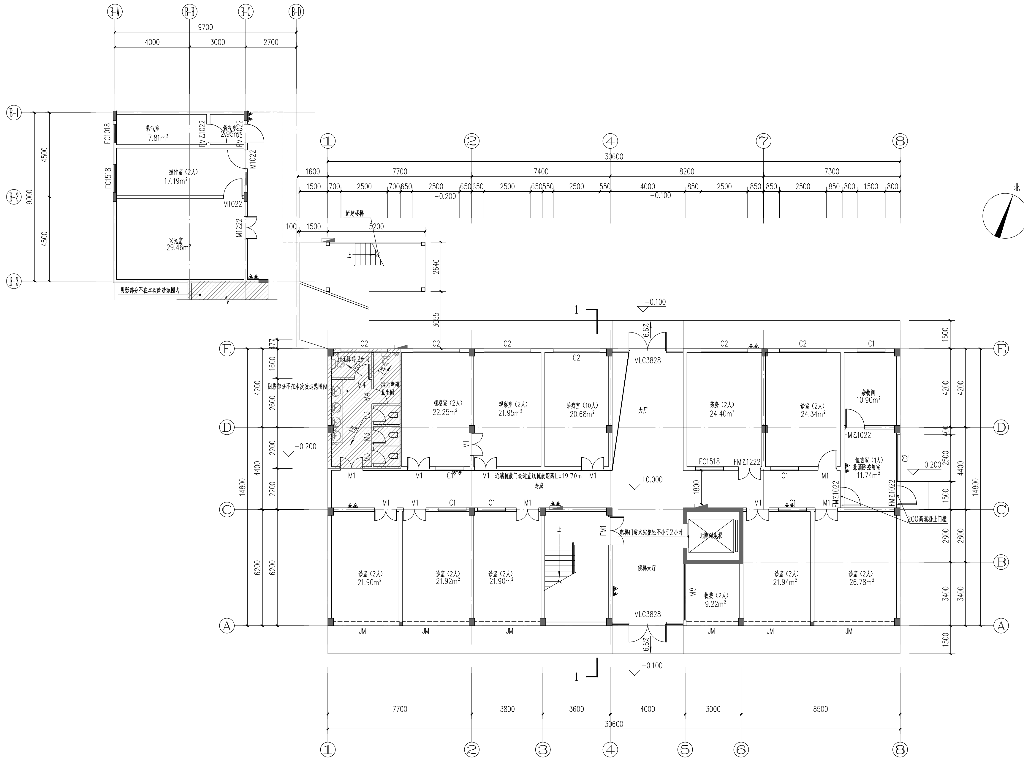
B、C栋首层改造平面图 1:100
