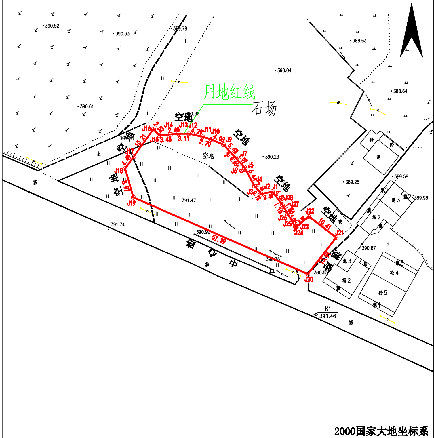
连州市小城镇（圩镇）人居环境治理工程（西江镇农贸市场停车场项目）规划用地红线图
