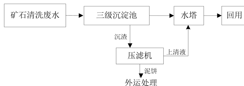
图 4-3 本项目废水回用处理系统工艺流程图
