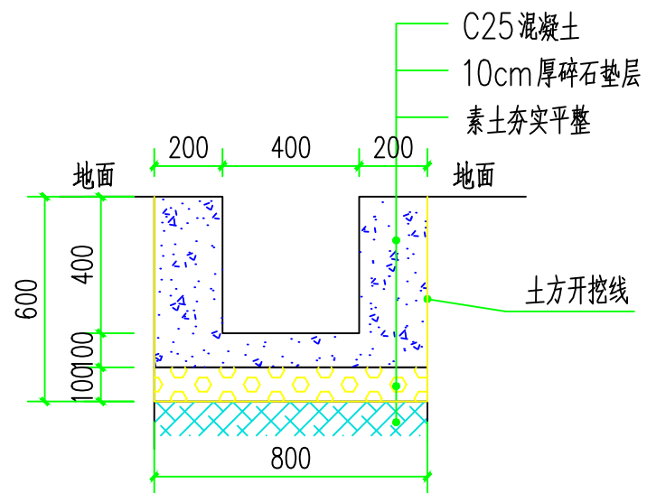
1 新建排水沟大样图 1:20 共: 131m
